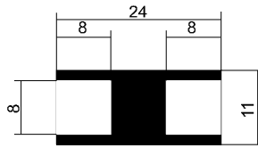
C35.5.121 Mittelstütze
